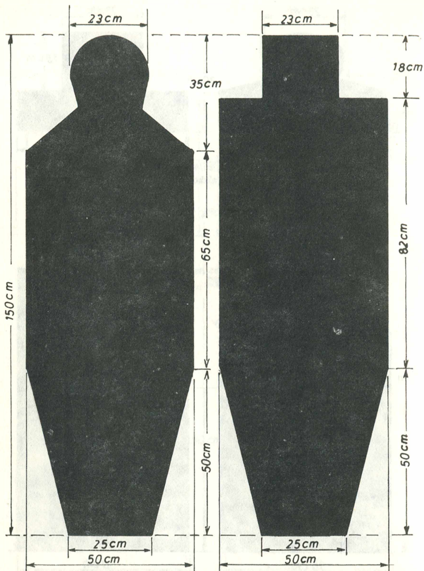
8. sz. céltábla Futóalakok
