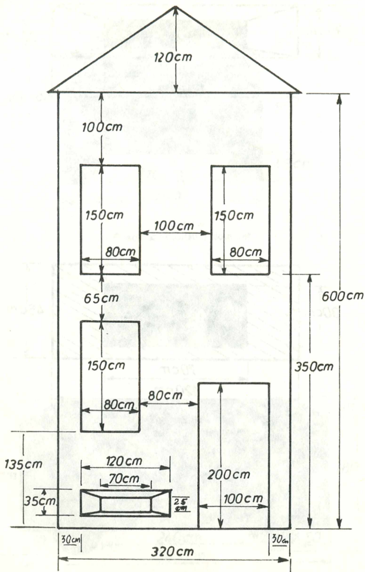
17. sz. céltábla Épületelem
