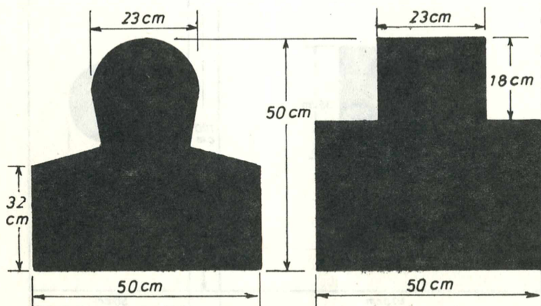
6. sz. céltábla Mellalakok
