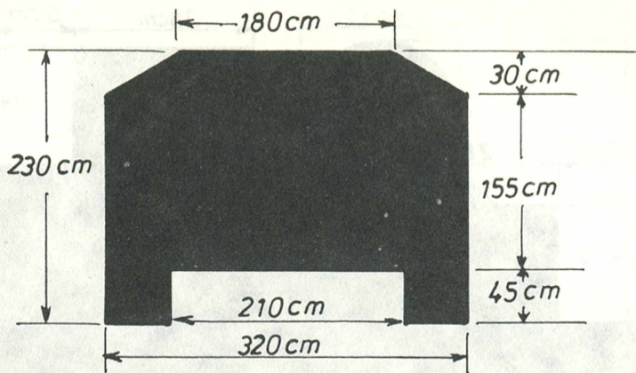
13. sz. céltábla Páncélozott szállítójármű előlnézet
