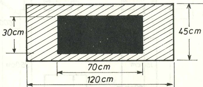
16. sz. céltábla Lőrésék
