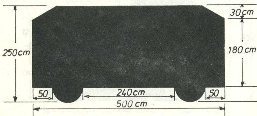
14. sz. céltábla Gépjármű oldalnézet
