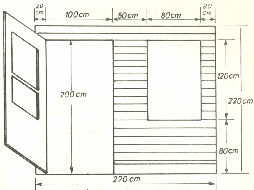
Épületelem ajtó-ablak makett
