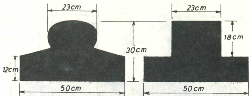
5. sz. céltábla Fejalakok
