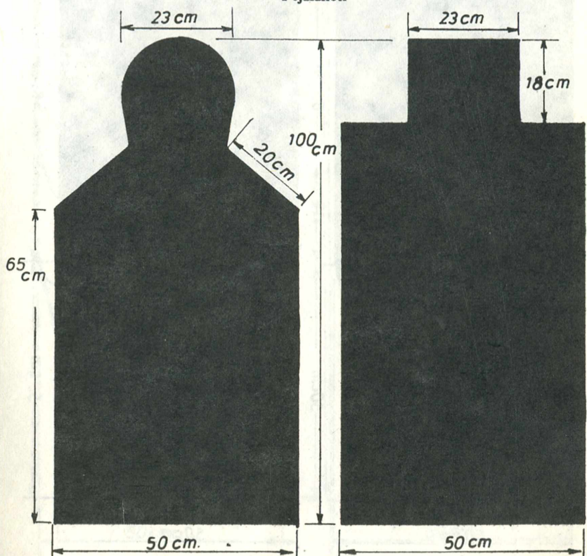
7. sz. céltábla Csípőalakok
